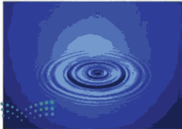
الشكل ١ الأمواج تنقل الطاقة عبر الماء كما تنقل الأمواج الزلزالية الطاقة عبر الأرض.
