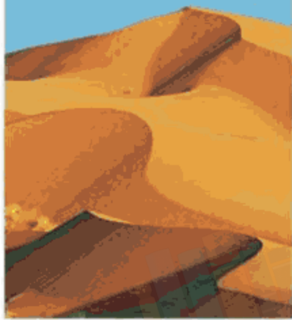
الشكل ٢٧ نقل الرياح للرمال يكوّن كتيباً رملية. ومع حركة الرياح فوق الكتيب الرملي، تتحرك رماله وتسقط فوق الجهة الأخرى. وبهذه الطريقة يقوم الكتيب بالهجرة فوق الأرض.
